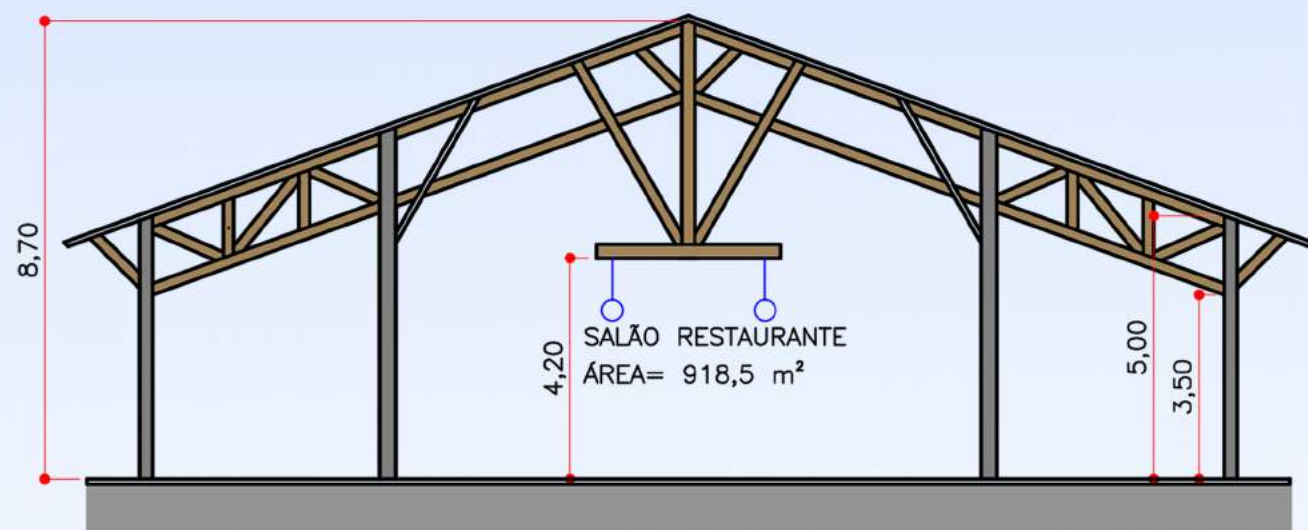
CORTE ESQUEMÁTICO COM AS ALTURAS. PÉ DIREITO SALÃO
